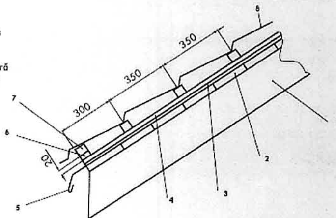
Detaliu streășină și schema montării șipcii orizontale:
